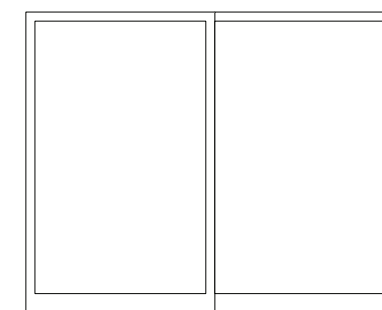
BSD2 25X20DM BALKONGDØR - HEVE/SKYVEDØR ANTALL: 2 STK GUSTAV BYES VEI 4 OG 14 BRYSTNING 138 MM INGEN SPROSSER
