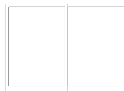
BSD1 26,5X19DM BALKONGDØR - HEVE/SKYVEDØR ANTALL: 39 STK BRYSTNING 138 MM INGEN SPROSSER
